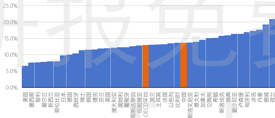
图 1：中国与 OECD 国家实收口径宏观税负比较
